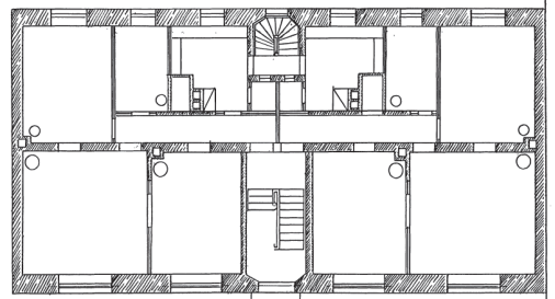
Stueplan
