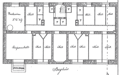
Kælderplan
